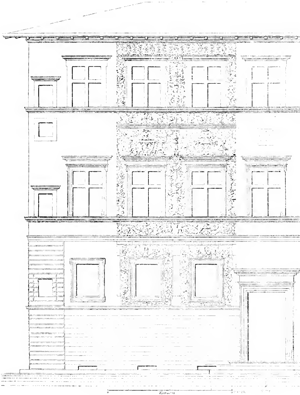
Zeit der Fassade des kleinen Palazzo Corsi in Florenz.
